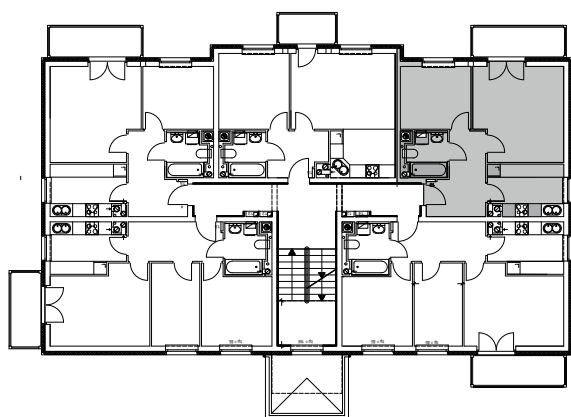
PIERWSZE PIĘTRO
